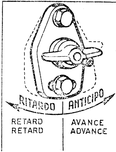
Fig. 6 - REGISTRAZIONE DELLA FINE POMPATA. RECLAGE DE FIN POMPAGE. SETTING END OF PUMP ACTION.
